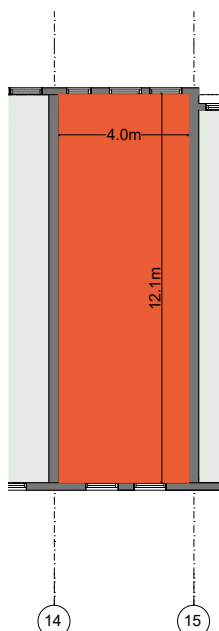
1 e verdieping
