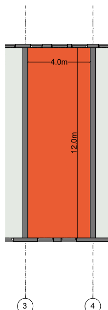
1e verdieping
