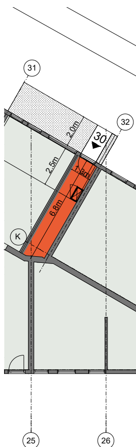
Begane grond
