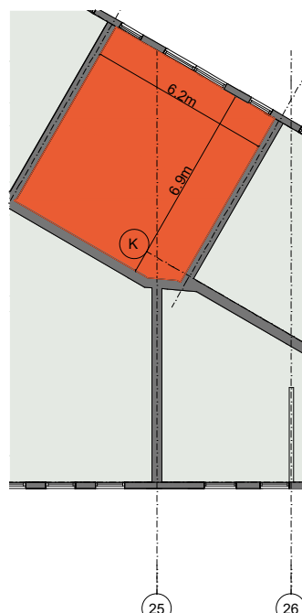
2 e verdieping
