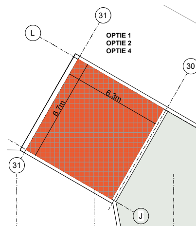
Dakoppervlakte
