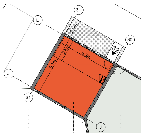
Begane grond
